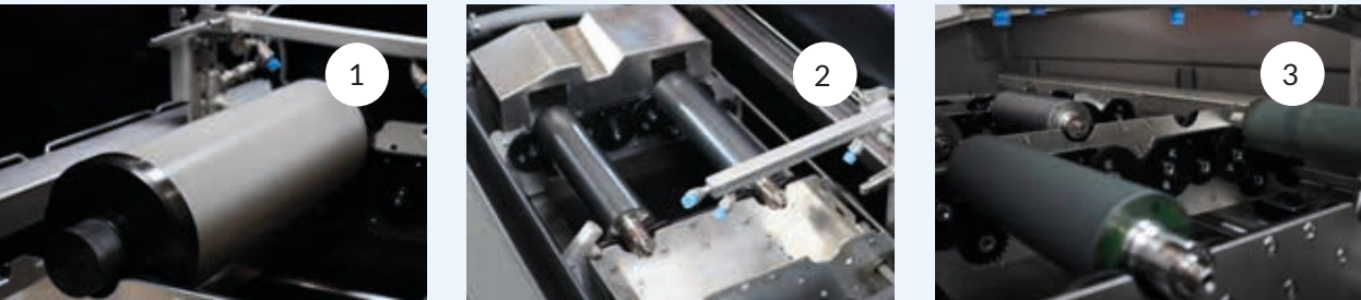
1: Para las mangas anilox, se puede hacer un adaptador según las medidas específicas del anilox. 2: Para los rodillos anilox, las unidades pueden fabricarse con cubiertas de engranajes para proteger los ejes. 3: Al añadir estaciones de tracción adicionales en las unidades FW 993, puede lavar hasta 9 aniloxes en un solo ciclo de limpieza.
