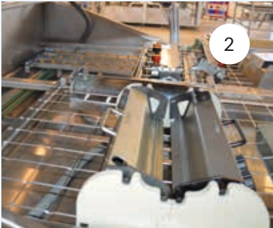
1: Soporte de cámara para cámaras Gallus, 2: Soporte de cámara para cámara Nilpeter, 3: Se pueden colocar boquillas giratorias en la rejilla para la limpieza de los cubos.
