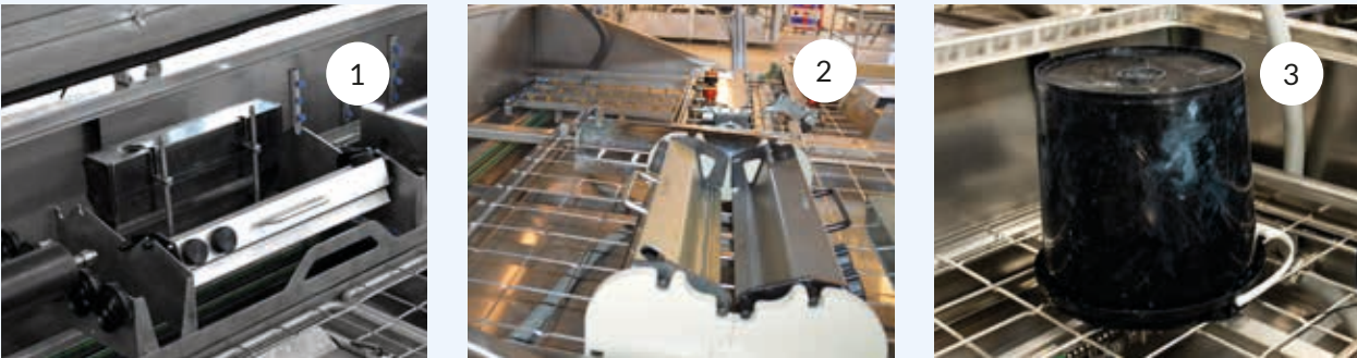
1: Kammerhalter für Galluskammern, 2: Kammerhalter für Nilpeter-Kammer, 3: Zum Reinigen von Eimern können rotierende Düsen auf das Gitter gestellt werden.
