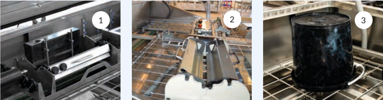
1: Soporte de cámara para cámaras Gallus, 2: Soporte de cámara para cámara Nilpeter, 3: Se pueden colocar boquillas giratorias en la rejilla para la limpieza de los cubos.
