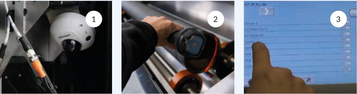
1: Cámara: vea el proceso de limpieza en tiempo real en la pantalla. 2: Fácil acceso a los detalles de los anilox en la base de datos, ya sea mediante un lector de códigos de barras o una identificación automática de anilox (RFID). 3: Los datos de limpieza de cada anilox se registran en la base de datos.
